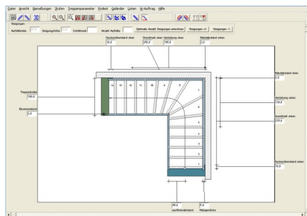
Schody jednozabiegowe - Rzut z góry
