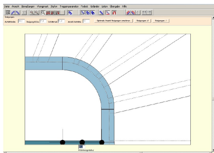
Podgląd szczegółowy krzywulca
